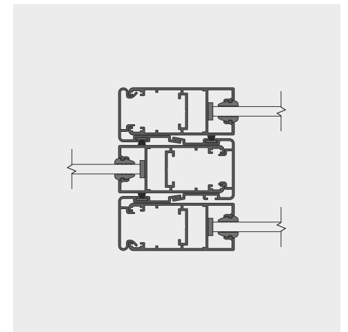
29mm FLYMESH
