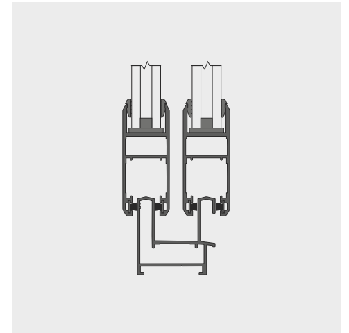
27mm DGU
