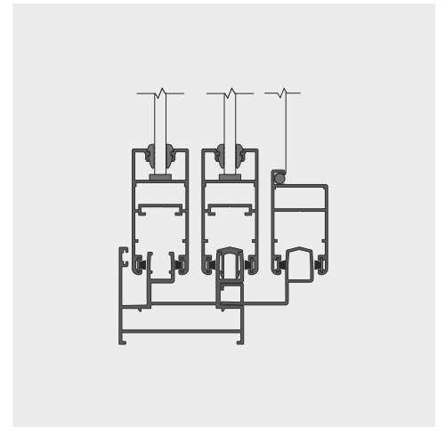
29mm FLYMESH
