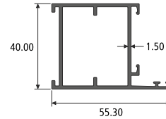
DOOR FRAME SECTION NO. : 819022 Weight / Mtr : 0.783
