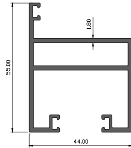
DOOR PROFILE
